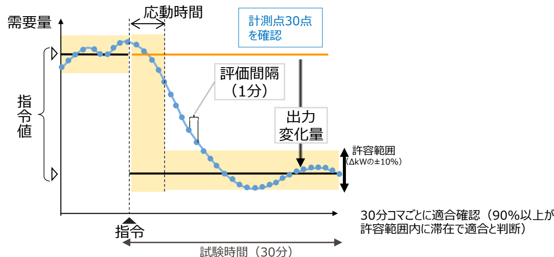
【出力変化量のイメージ(DSR等の例)】
