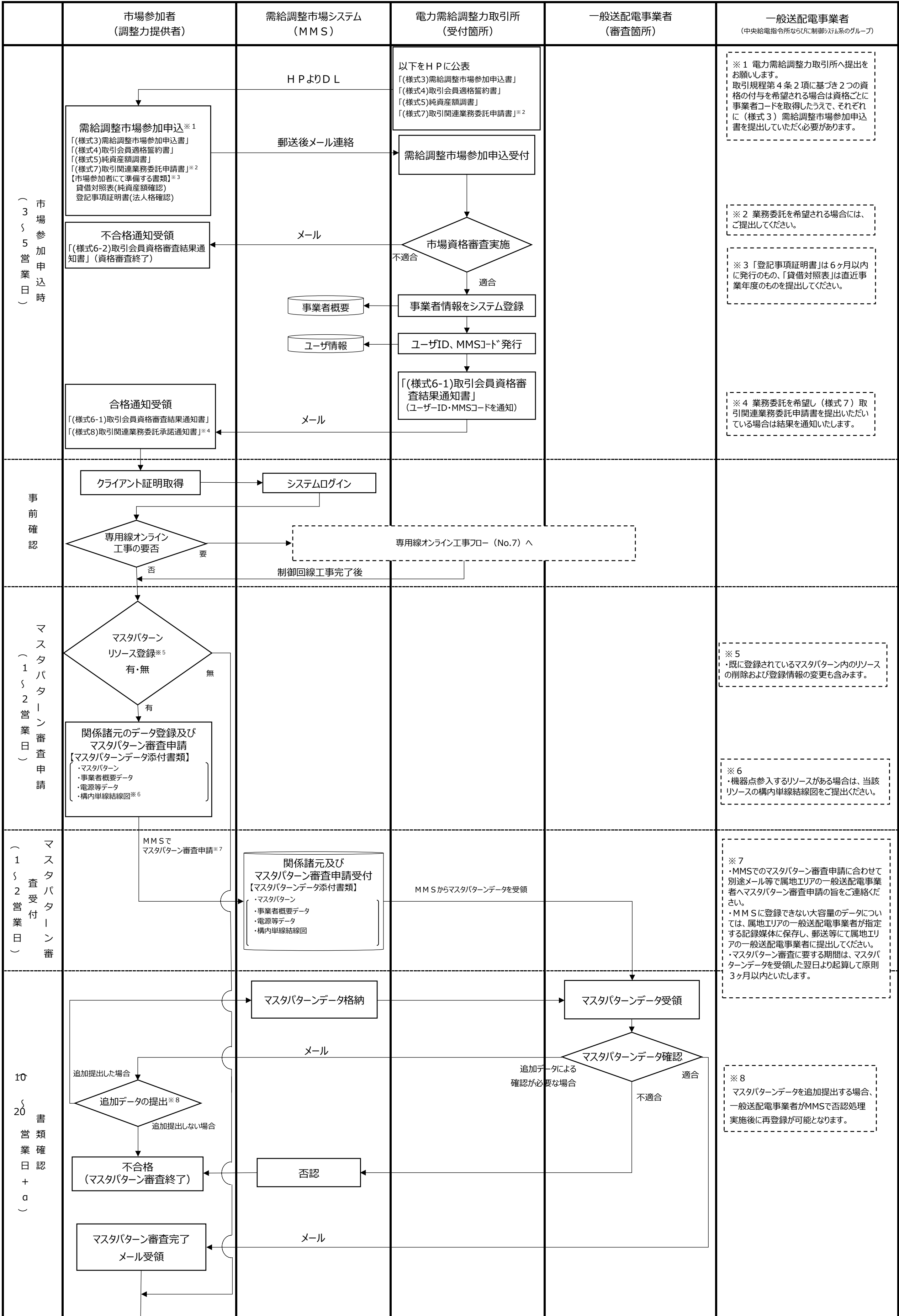
○需給調整市場の事前審査に伴う業務フロー（各リスト・パターン：発電機リスト・パターン）【一次調整力】
